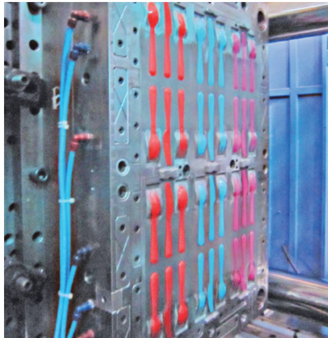
IKEA-36穴3色成型2套 IKEA-36-cavity 3-color Molding 2 Set
